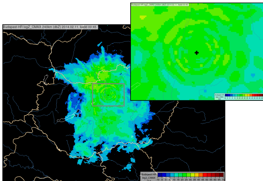
17. ábra. A 2014. 02. 11. 00.45 UTC-kor a budapesti radar által mért reflektivitási mező.
