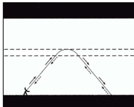
21. ábra. Anaprop terjedés.
