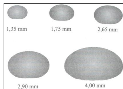
6. ábra. Az esőcsepp alakja méretének függvényében.
