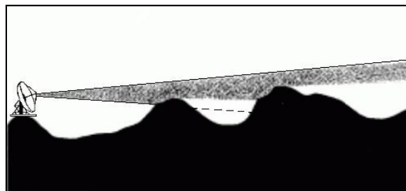
22. ábra. Nyaláb blokkolás.
