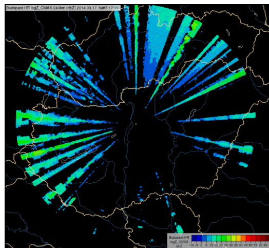
18. ábra. WLAN zavarok hatása a budapesti radar mérésére egy extrém esetben. A képen látható jeleket egyedül WLAN zavarok okozzák, ebben az időpontban csapadék nem volt a térségben.
