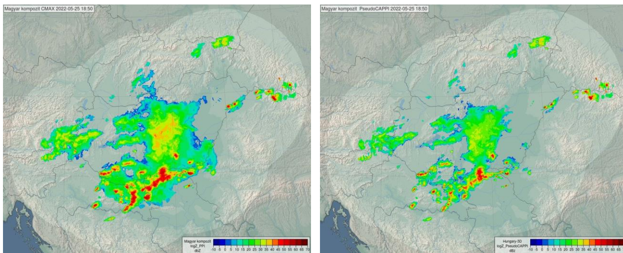
9. ábra. 2022. 05. 25-én készült Oszlopmaximum és PseudoCAPPI kompozit reflektivitás képek. Oszlopmaximum esetén gyakran nagyobb reflektivitás értékek adódnak, illetve jóval több a gyenge jel, amik többnyire a talajt el nem érő magasabb rétegekből származnak.
