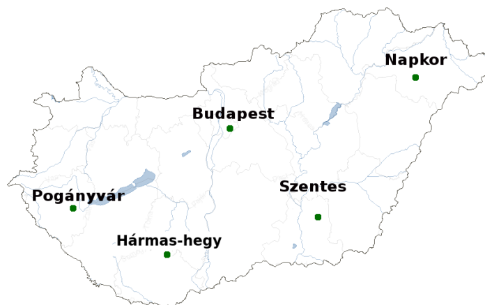
2. ábra. Az Országos Meteorológiai Szolgálat időjárási radarhálózatának tagjai.
